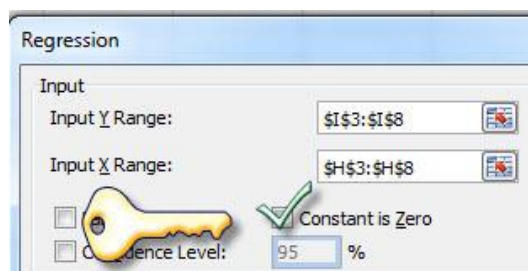
Фигура 1. Регресионно извеждане на коефициент „бета”
